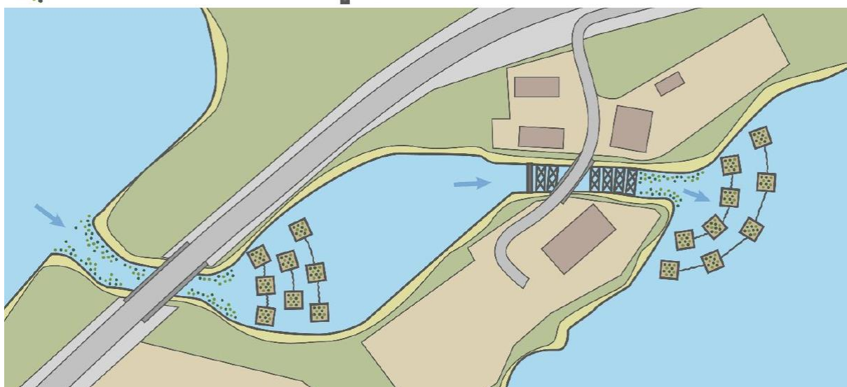
Rysunek 3 Wizualizacja projektu oczyszczania wód na dopływie z jeziora Sunowo do Jeziora Ełckiego (źródło: Badania wody oraz pomiary hydrologiczne rzeki Ełk oraz dopływu z jeziora Sunowo pod kątem oceny źródeł zanieczyszczeń wraz ze sporządzeniem projektu koncepcyjnego ochrony wód płynących, 2020).
