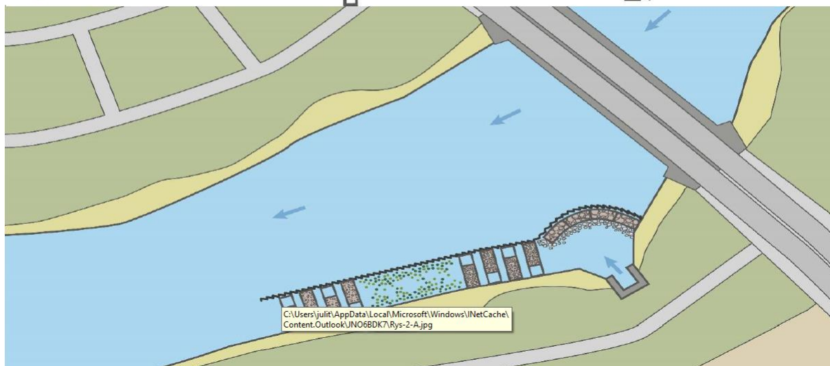
Rysunek 2 Wizualizacja metody podczyszczania wody opadowej odprowadzanej siecią kanalizacji deszczowej bezpośrednio do rzeki ze strefą mineralno-roślinną na przykładzie wylotu kanalizacji deszczowej przy ul. Wojska Polskiego (źródło: Badania wody oraz pomiary hydrologiczne rzeki Ełk oraz dopływu z jeziora Sunowo pod kątem oceny źródeł zanieczyszczeń wraz ze sporządzeniem projektu koncepcyjnego ochrony wód płynących, 2020).
