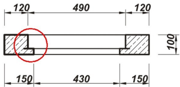
Rysunek nr 2 – Rama typu lekkiego
