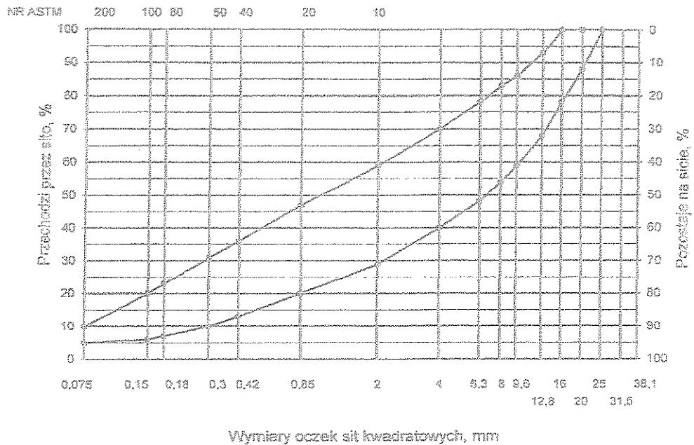
Rys. 1. Krzywe graniczne uziarnienia mieszanki mineralnej BA od 0 do 20 mm do warstwy ściernalnej nawierzchni drogi o obciążeniu ruchem dla KRI lub KR2
