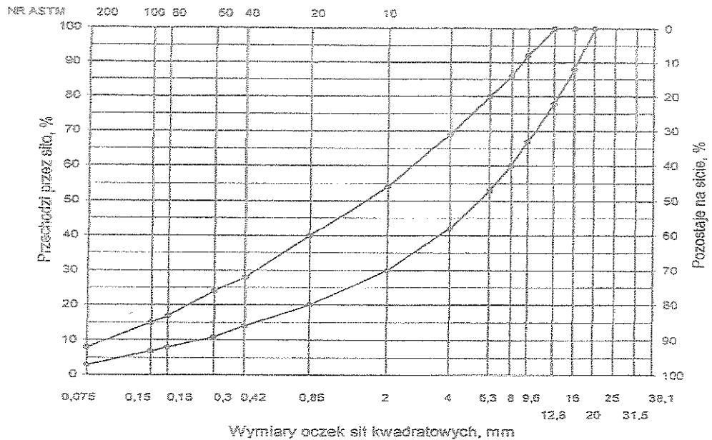
Rys. 9. Krzywe graniczne uziarnienia mieszanki mineralnej BA od 0 do 16 mm do warstwy wiążącej, wyrównawczej i wzmacniającej nawierzchni drogi o obciążeniu ruchem KRI lub KR2
