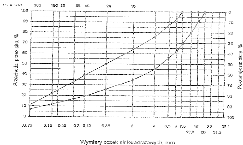
Rys. 2. Krzywe graniczne uziarnienia mieszanki mineralnej BA od 0 do 16mm. od 0 do 12,8 mm do warstwy ścieralnej nawierzchni drogi o obciążeniu ruchem KRI lub KR2
