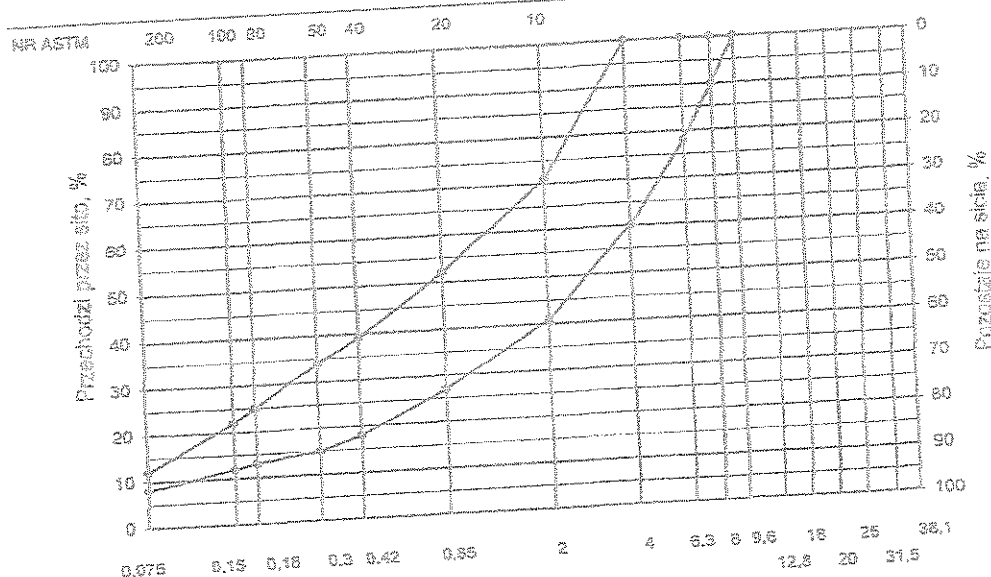
Rys. 3. Krzywe graniczne uziarnienia mieszanki mineralnej BA od 0 do 8mm. od 0 do 6,3 mm do warstwy ścieralnej nawierzchni drogi o obciążeniu ruchem nawierzchni drogi o obciążeniu ruchem KRI lub KR2
