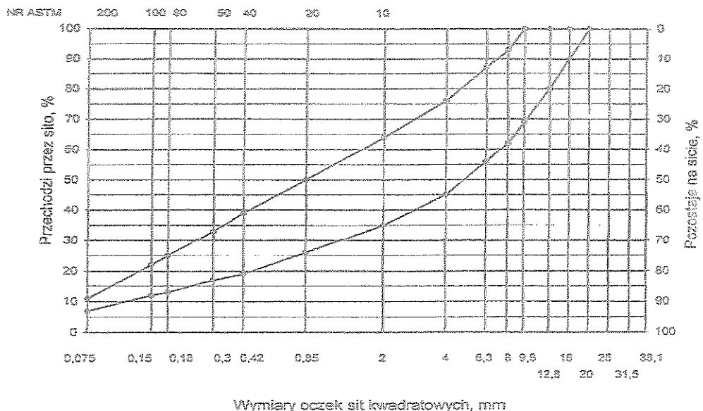
Rys. 2. Krzywe graniczne uziarnienia mieszanki mineralnej BA od 0 do 16mm, od 0 do 12,8 mm do warstwy ściernalnej nawierzchni drogi o obciążeniu ruchem KRI lub KR2
