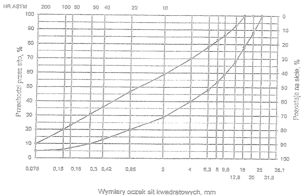
Rys. 1. Krzywe graniczne uziarnienia mieszanki mineralnej BA od 0 do 20 mm do warstwy ścieralnej nawierzchni drogi o obciążeniu ruchem dla KRI lub KR2
