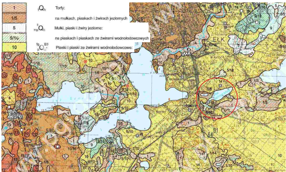
Rys.2.14. Szczegółowa mapa geologiczna, fragment arkusza nr 183 (czerwonym kołem oznaczony teren opracowania)
