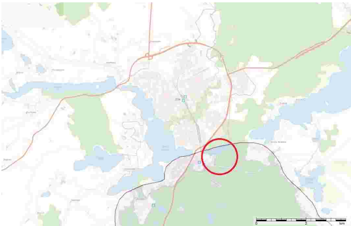
Rys. 2.20. Fragment mapy hydrogeologicznej Polski (czerwonym okręgiem oznaczony jest teren opracowania) (źródło: http://epsh.pgi.gov.pl/epsh/ )
