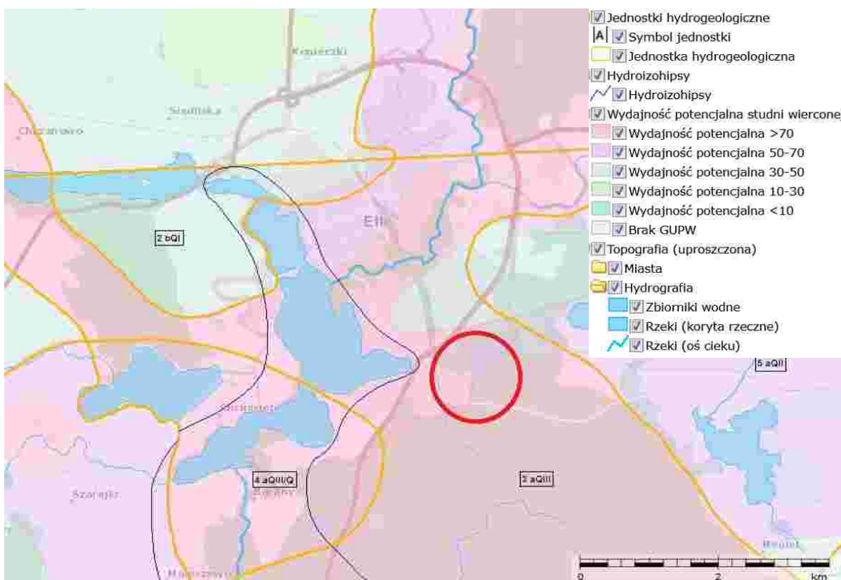
Rys. 2.21. Szczegółowa mapa hydrogeologiczna, fragment arkusza nr 183 (czerwonym kołem oznaczony teren opracowania)
